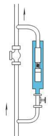
Рис. 3. Водоснабжение высотных зданий
